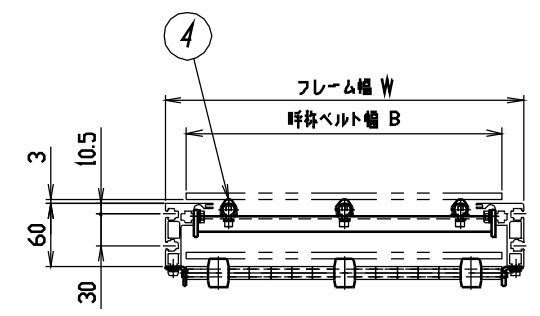
中間断面
