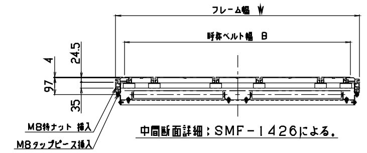
幅関係寸法
