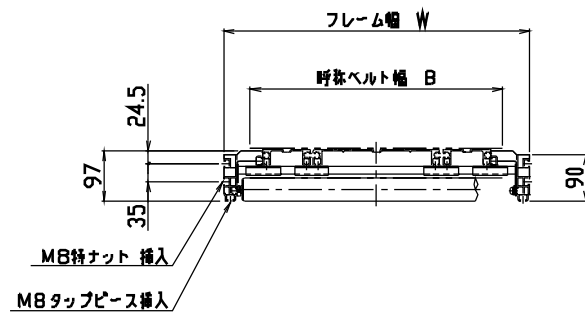
中間断面詳細: SMF-1421, 1422による
