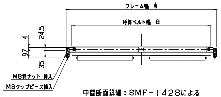
幅関係寸法
