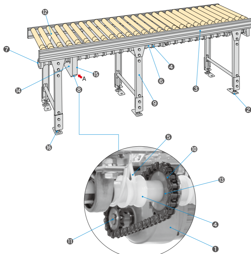
ドライブ内部(カバーを外した状態)
